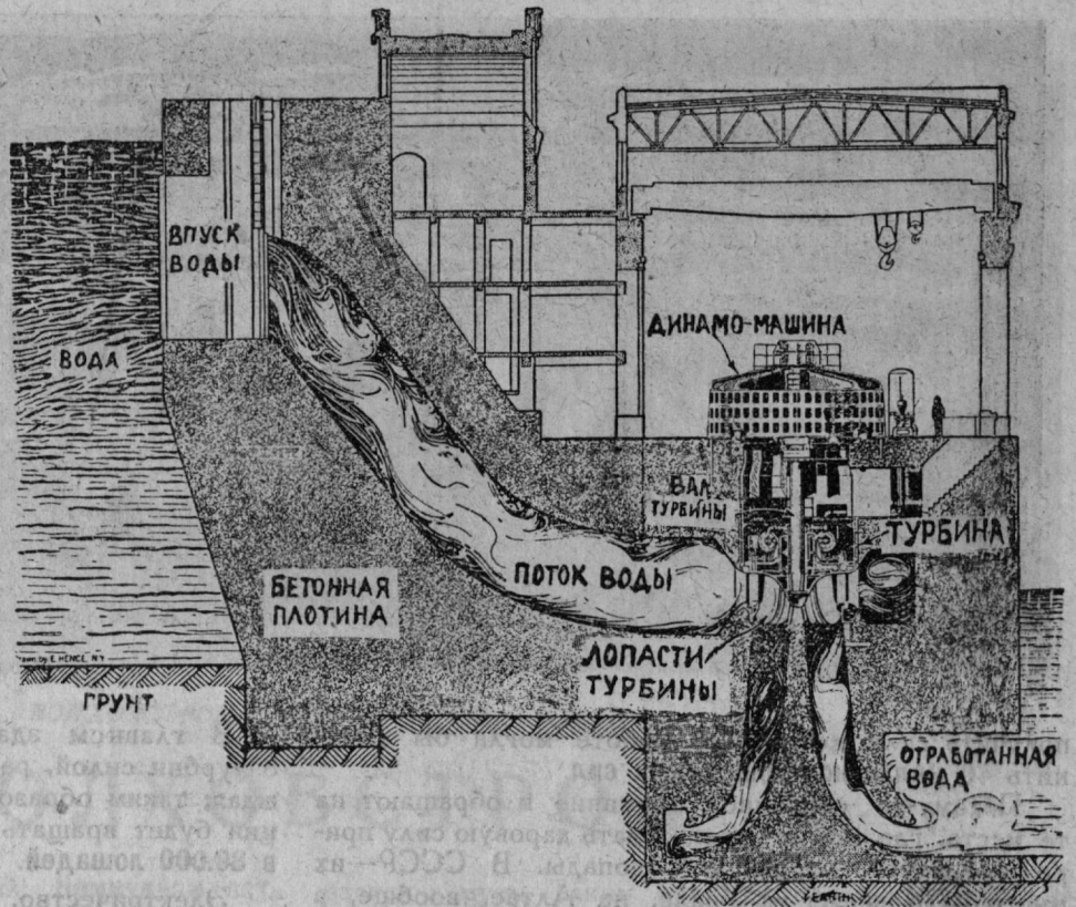
ВОЛХОВСТРОЙ. Разрез турбины.
